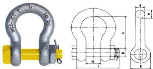
Скоба омегаобразная шплинт G2130
