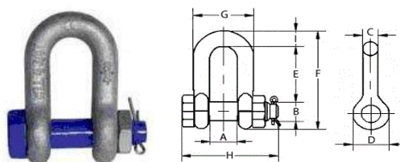
Скоба прямая шплинт G2150
