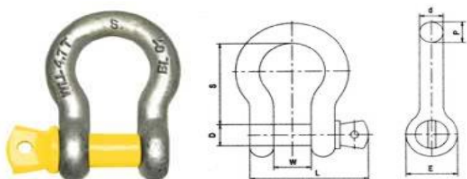
Скоба омегаобразная винтовая G209
