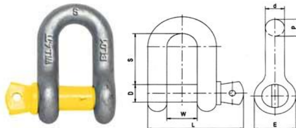
Скоба прямая винтовая G210
